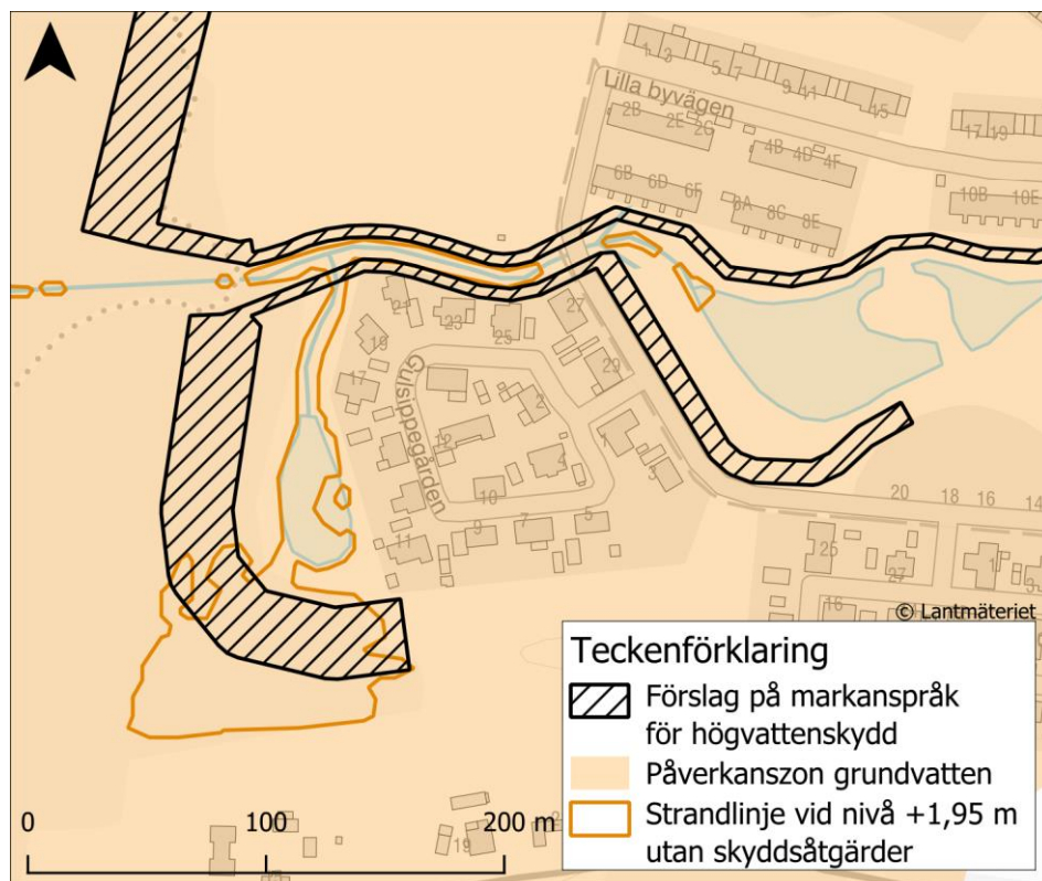
Figur 8-14 Påverkansområde för grundvatten samt läge för framtida strandlinje ifall inga skyddsåtgärder vidtas.
