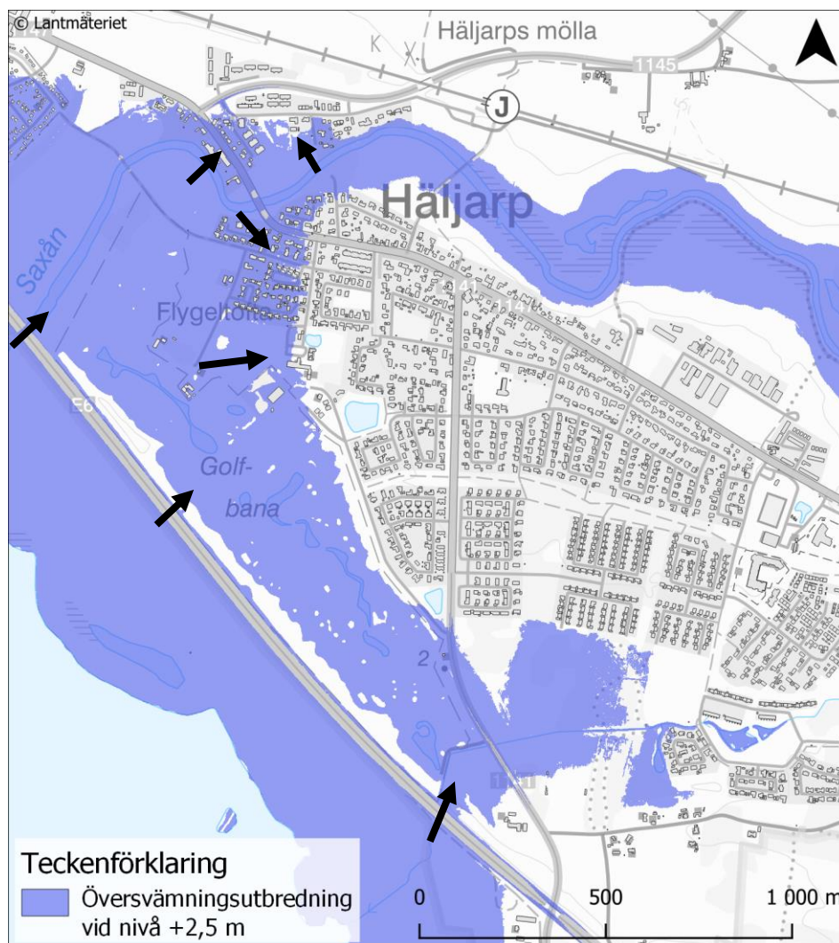
Figur 6-2 Översvämning vid vattennivå +2,5 m (RH2000), motsvarande ett 200-årshögvatten cirka år 2075. Inströmningsvägar är markerade med pilar.
