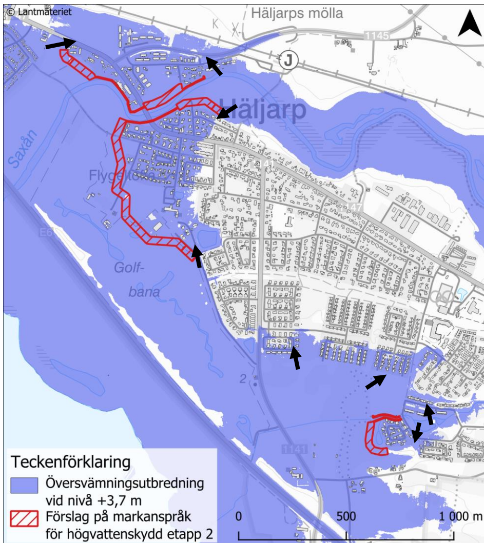
Figur 6-6 Översvämning vid högvattennivå +3,7 m (RH2000) med skydden från etapp 2 alternativ 1. Vattnet når över krönnivån på de föreslagna skydden, pilar markerar nya inströmningsvägar för vattnet.
