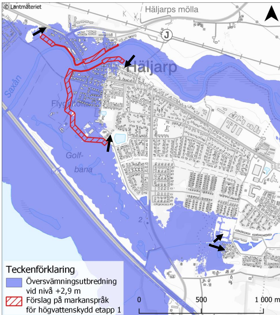
Figur 6-4 Översvämning vid högvattennivå +2,9 m (RH2000) med skydden från etapp 1 alternativ 1. Vattnet når över krönnivån på de föreslagna skydden, pilar markerar nya inströmningsvägar för vattnet.
